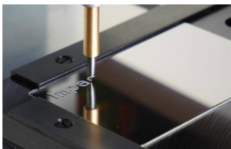
Pneumatischer Nadelpräger
